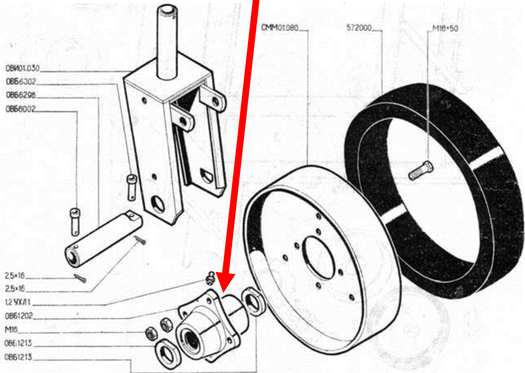
Рис. 6. Ход передний ОВИ 01.020. -12
